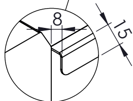
DETTAGLIO SCALA 1 : 2
